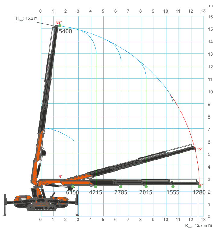
Hauptausleger
