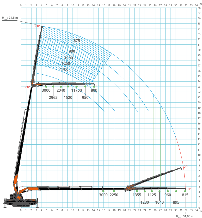
Hydraulischer Jib
