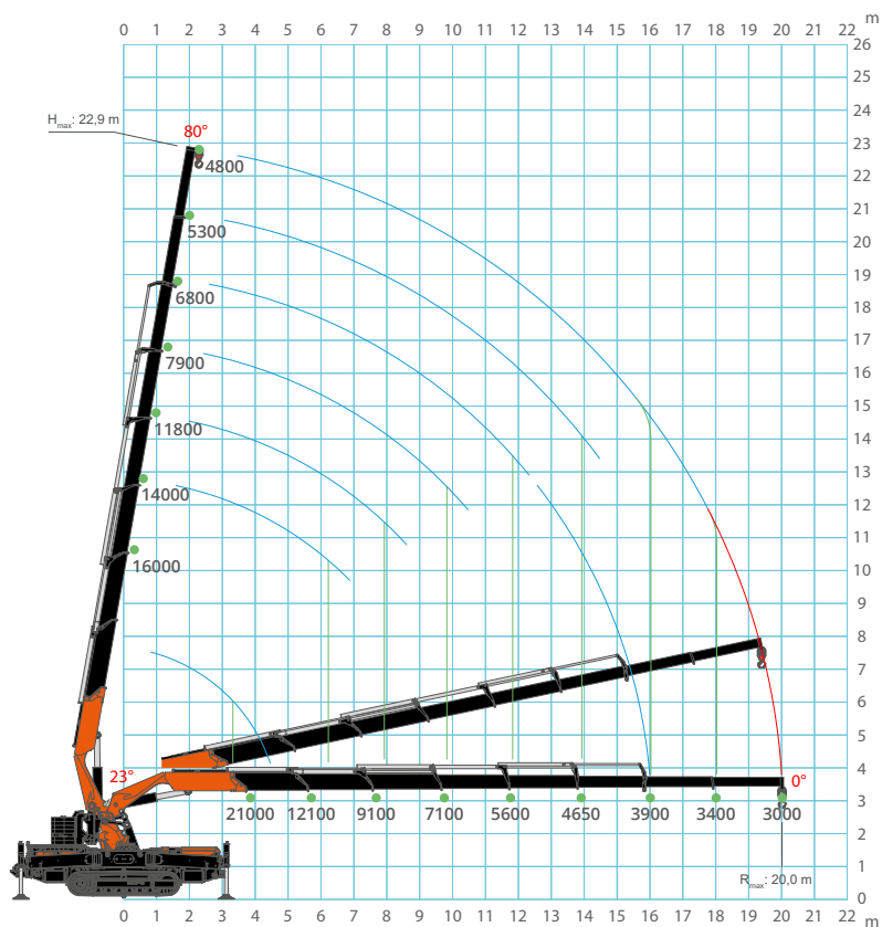
Hauptausleger
